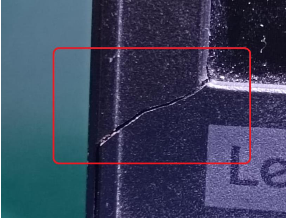
Cubierta de pantalla con deformado por golpe
