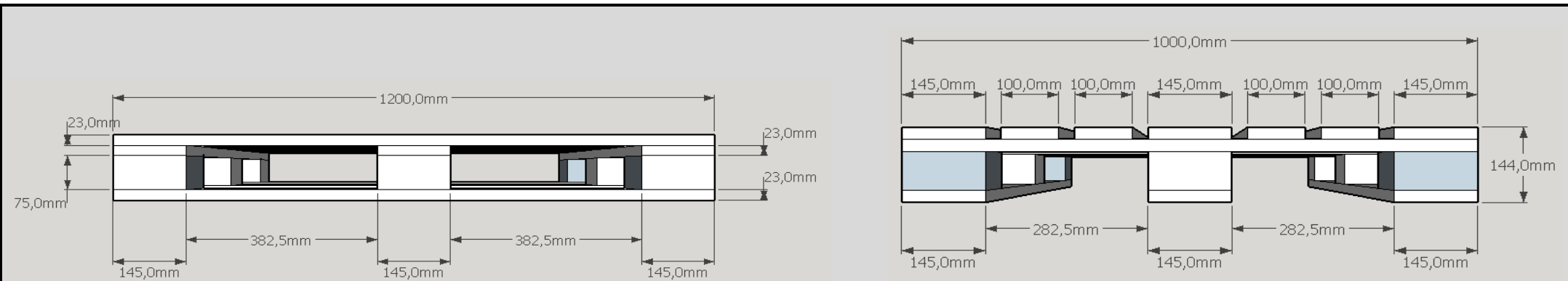
VISTA DE ELEVACIÓN
