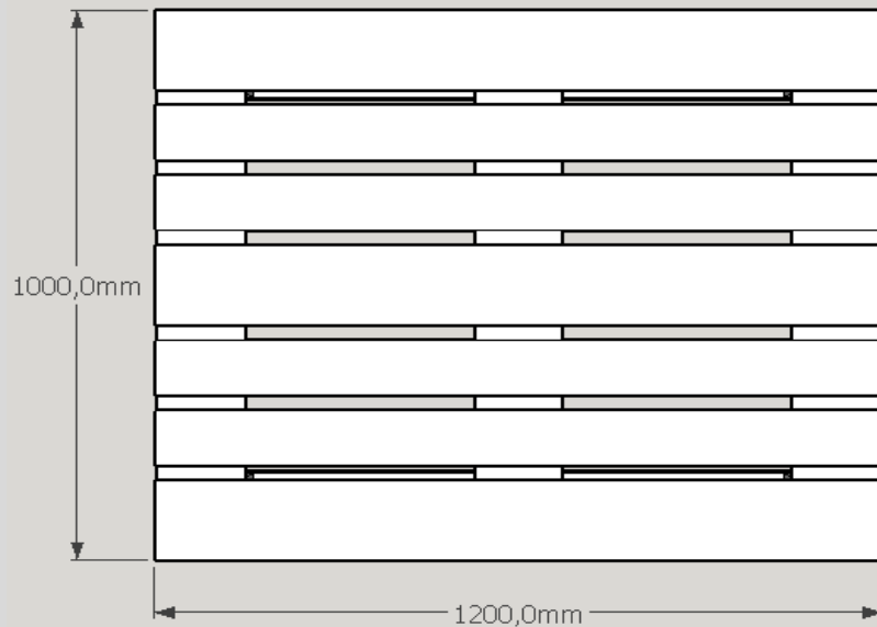
VISTA DE PLANTA
