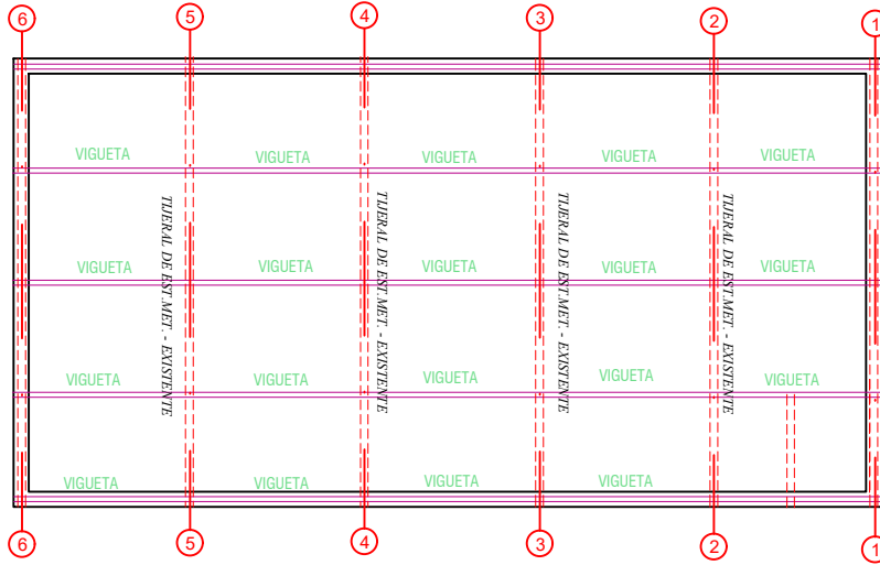
PLANTA COBERTURA ESC: 1/50
